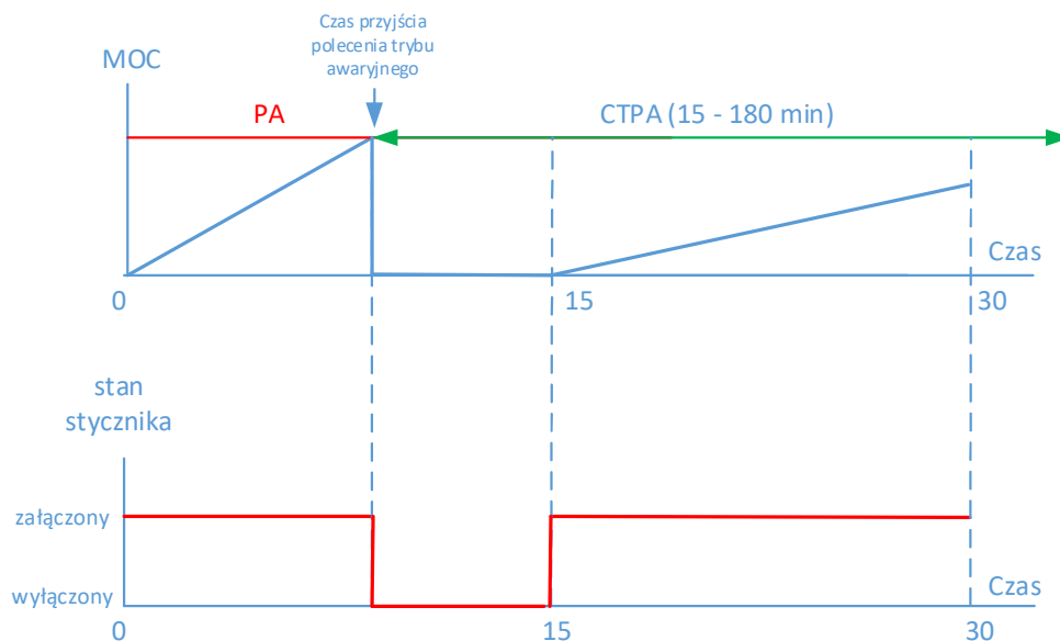
Rysunek 3: Ilustracja przykładu użycia dla trybu awaryjnego wraz ze stanem stycznika w przypadku gdy wartość mocy PA jest większa niż moc maksymalna wyliczona w ramach bieżącego 15-minutowego okresu całkowania (kwadrans 0-15) oraz gdy wartość mocy PA jest mniejsza niż moc maksymalna wyliczona w ramach bieżącego 15-minutowego okresu całkowania (kwadrans 15-30) .
